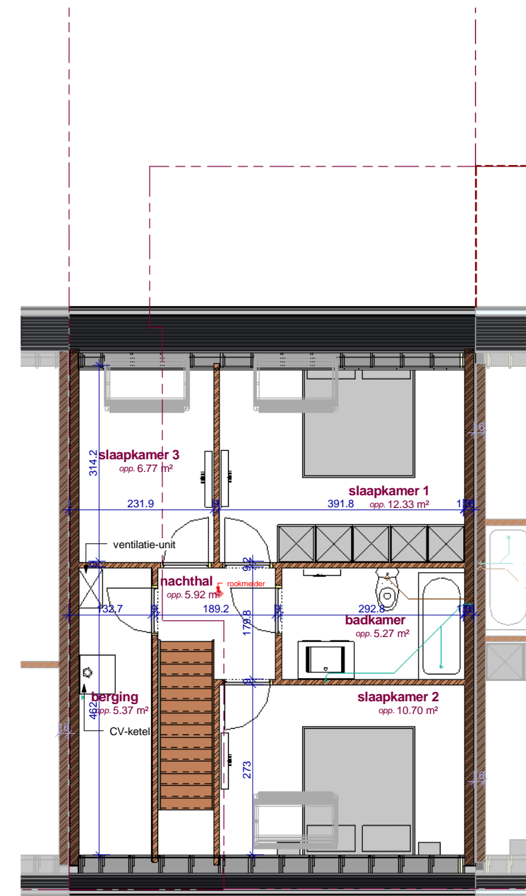
3 2de VERDIEPING 1 : 50
