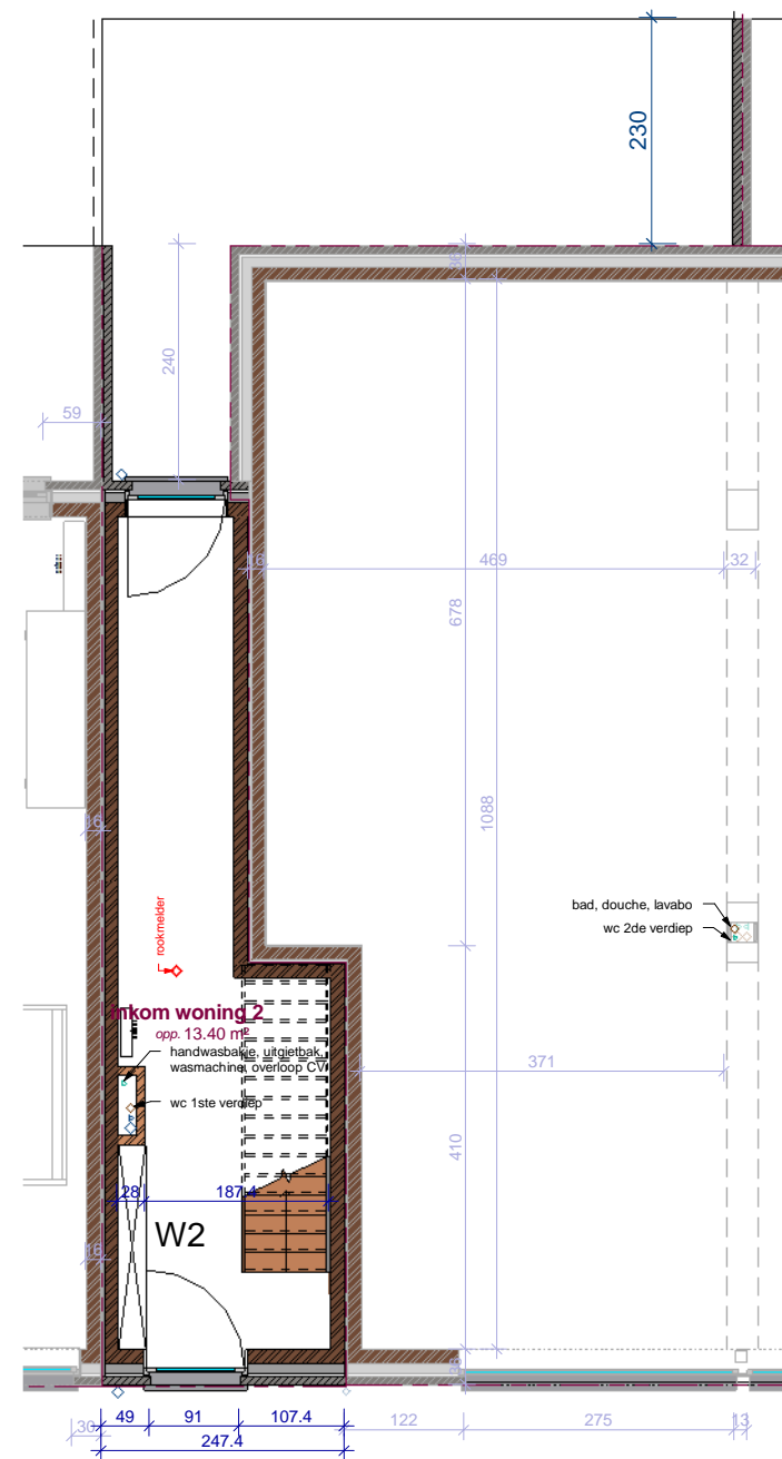
1 GRONDPLAN 1 : 50
