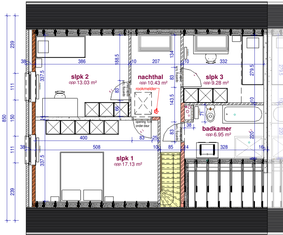
verdieping
