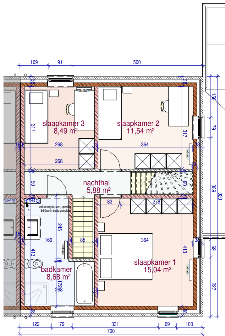
verdieping
