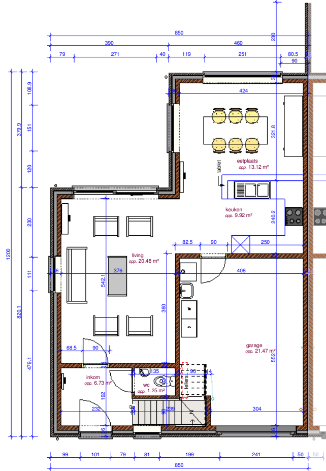
① Rez-de-chaussée lot 43 - R1R
