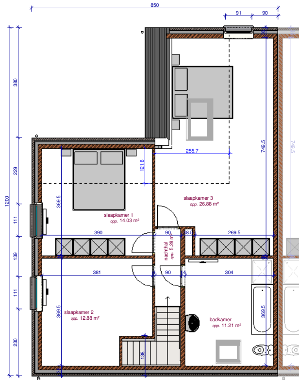
② étage lot 43 - R1R
