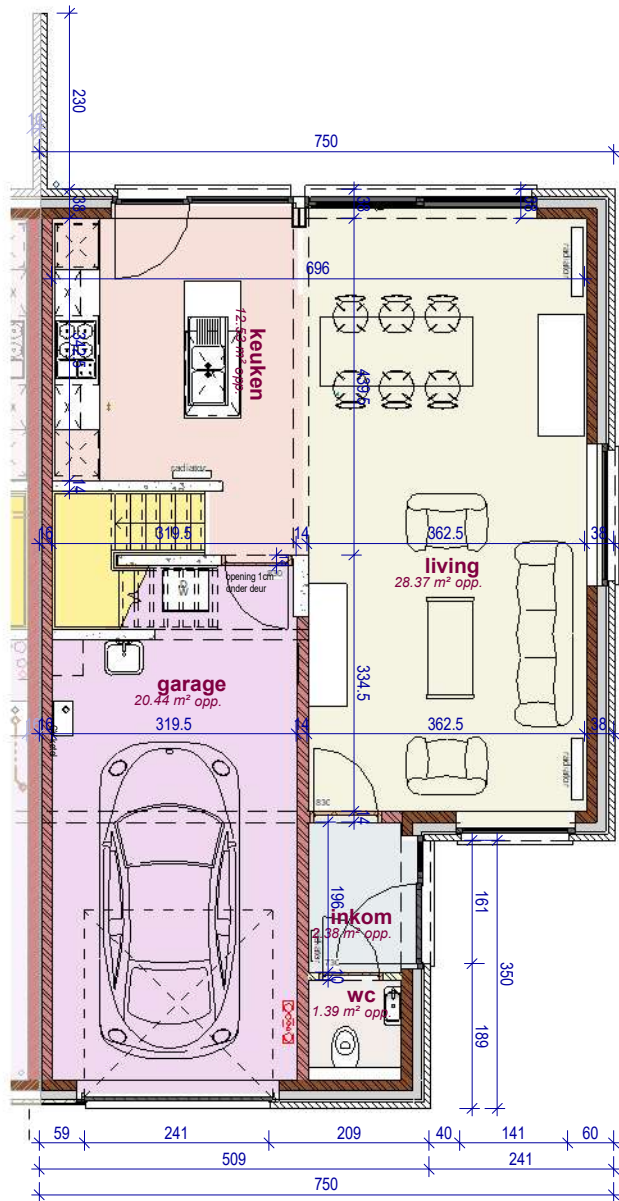
gelijkvloers 32 LL
