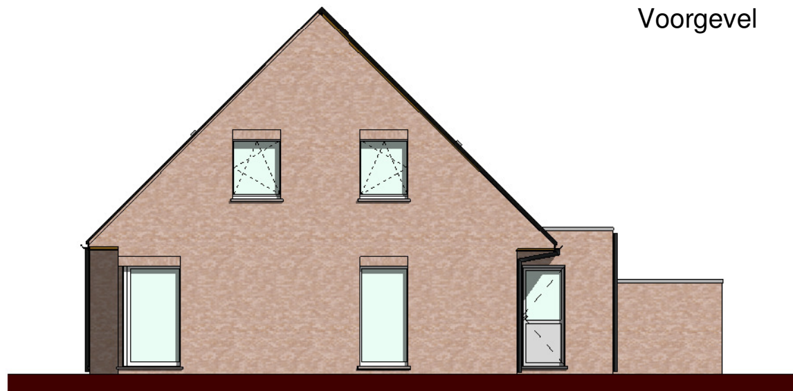
Gevel rechts
