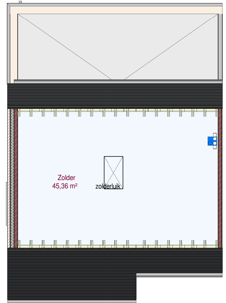
3 2e verdieping woning 1 LL 1 : 75
