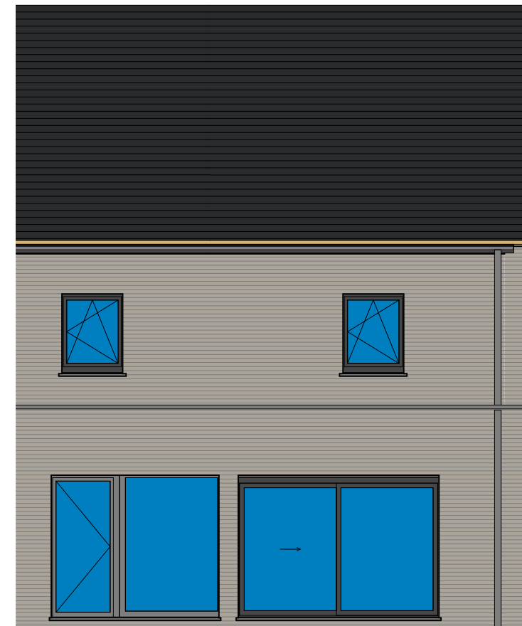
2 achtergevel woning 1 1 : 75
