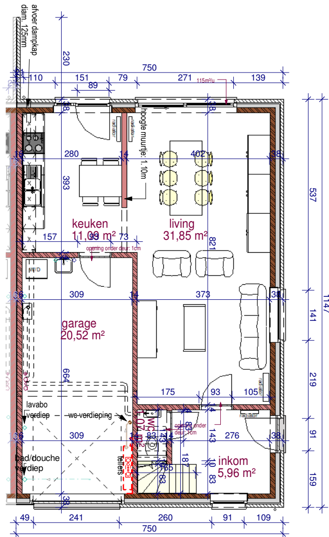
gelijkvloers
