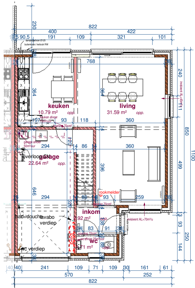
gelijkvloers
