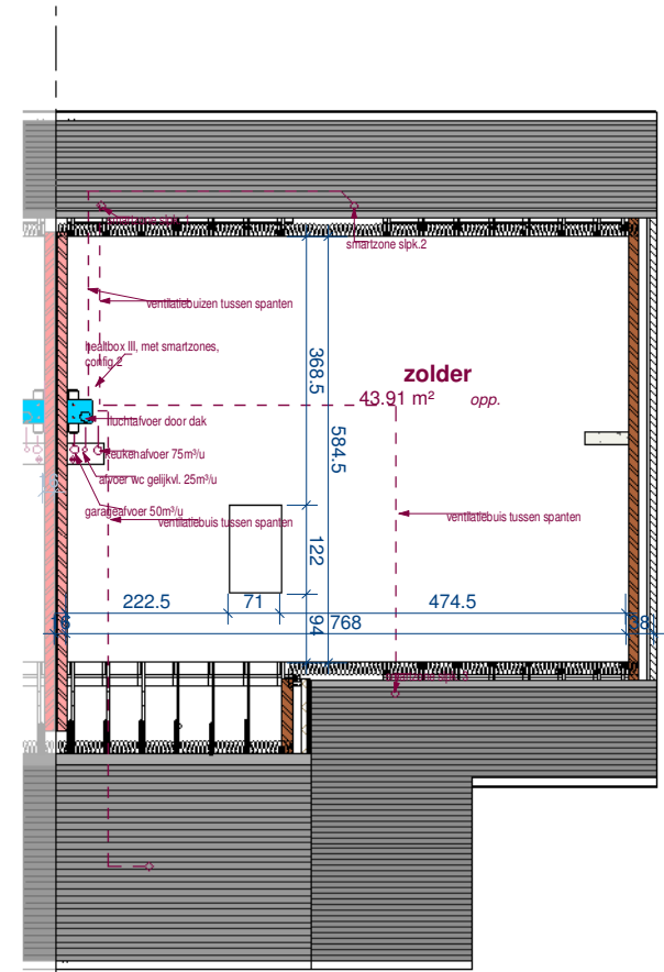
2de verdieping
