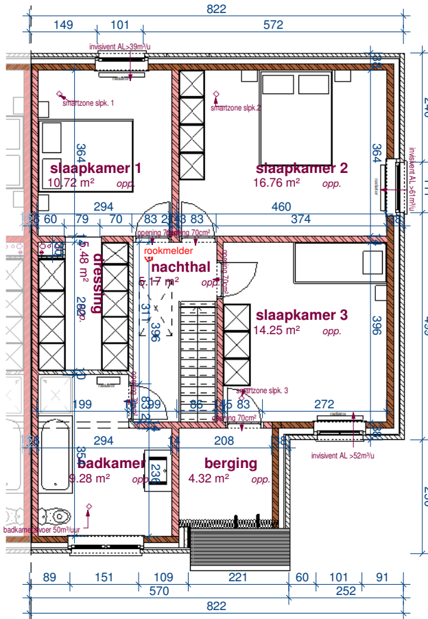
verdieping
