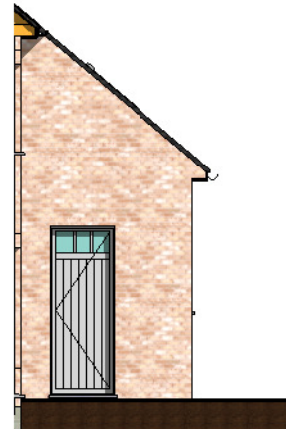
zijgevel links
