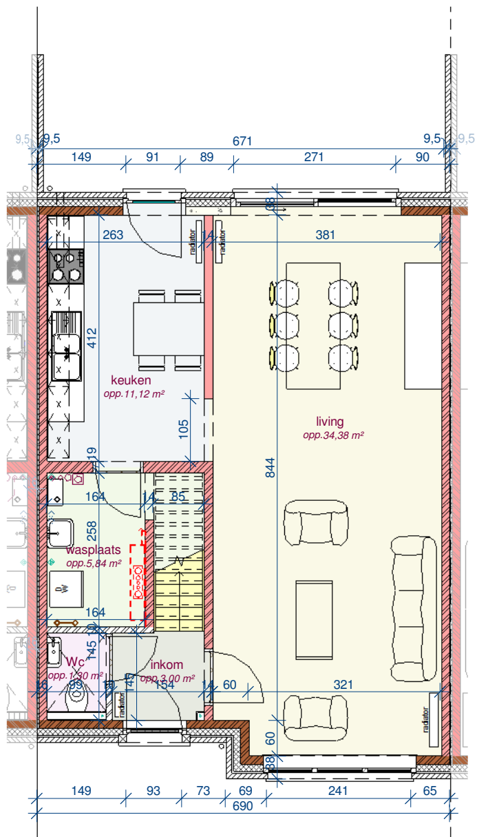
gelijkvloers
