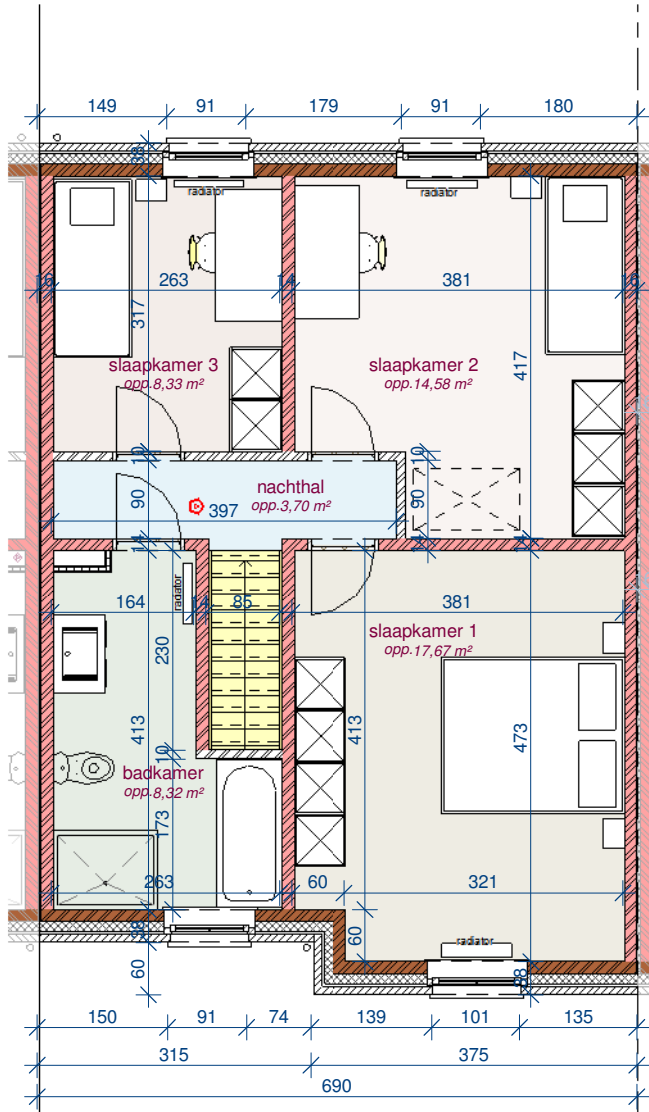
1ste verdieping
