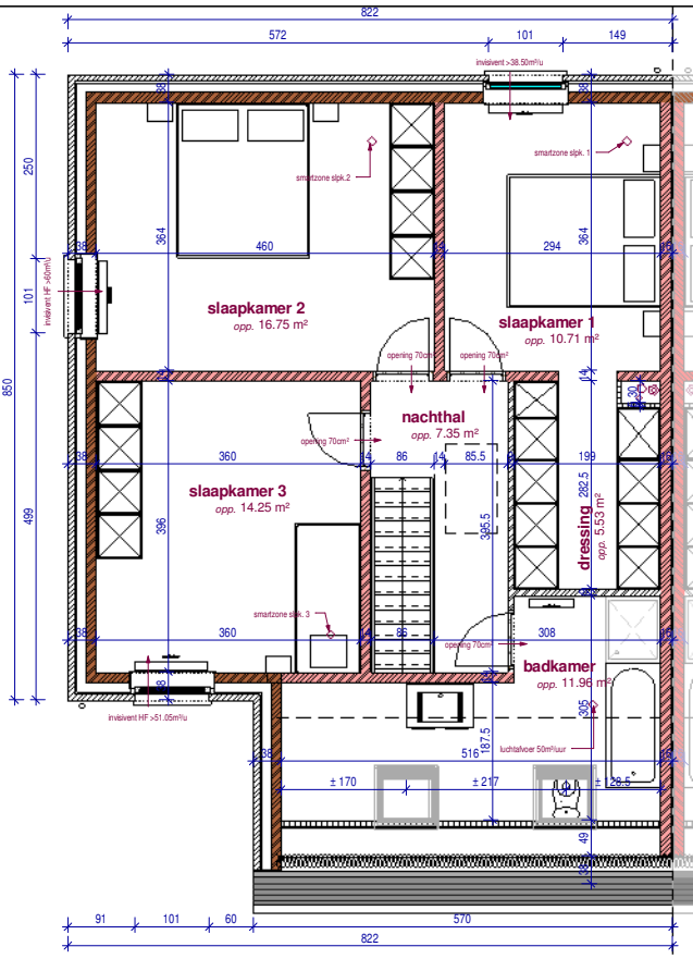
1ste verdieping
