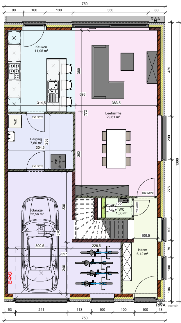
Gelijkvloers LL - lot 6
