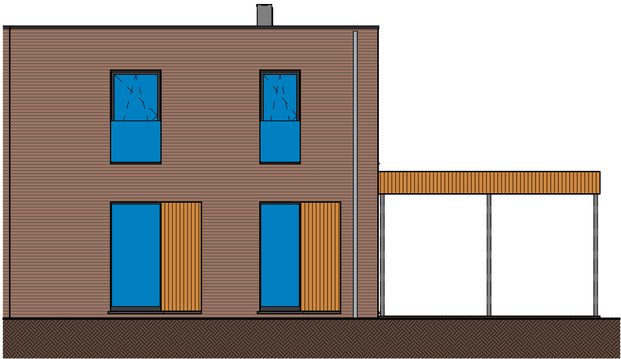
Voorgevel
