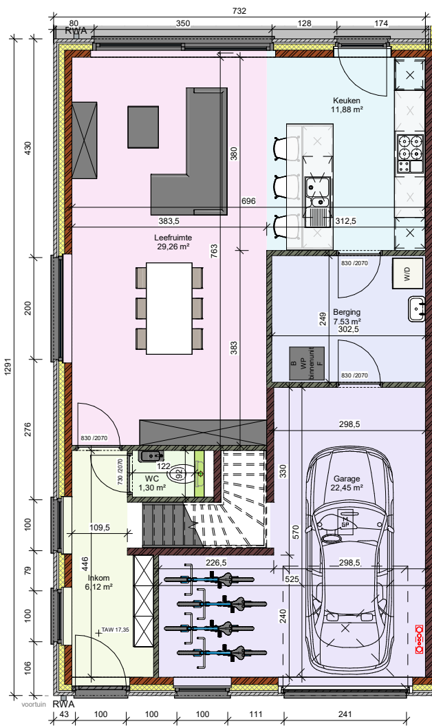
Gelijkvloers LL - lot 1
