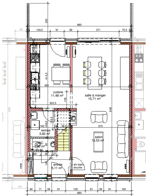
1 rez-de-chaussee 1 : 50
