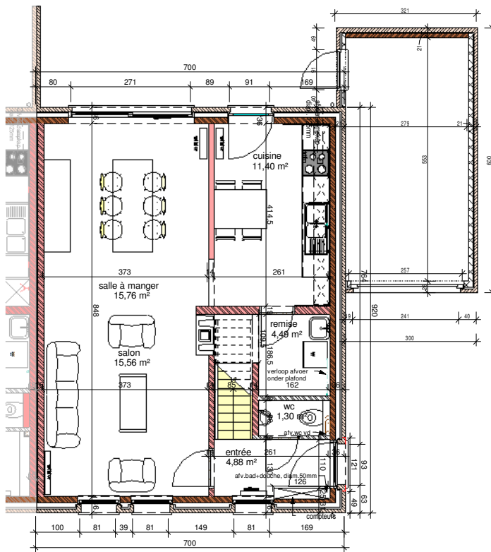
① rez-de-chaussee 1 : 50
