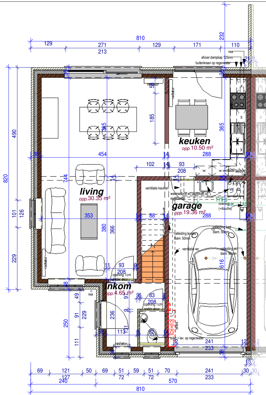
gelijkvloers
