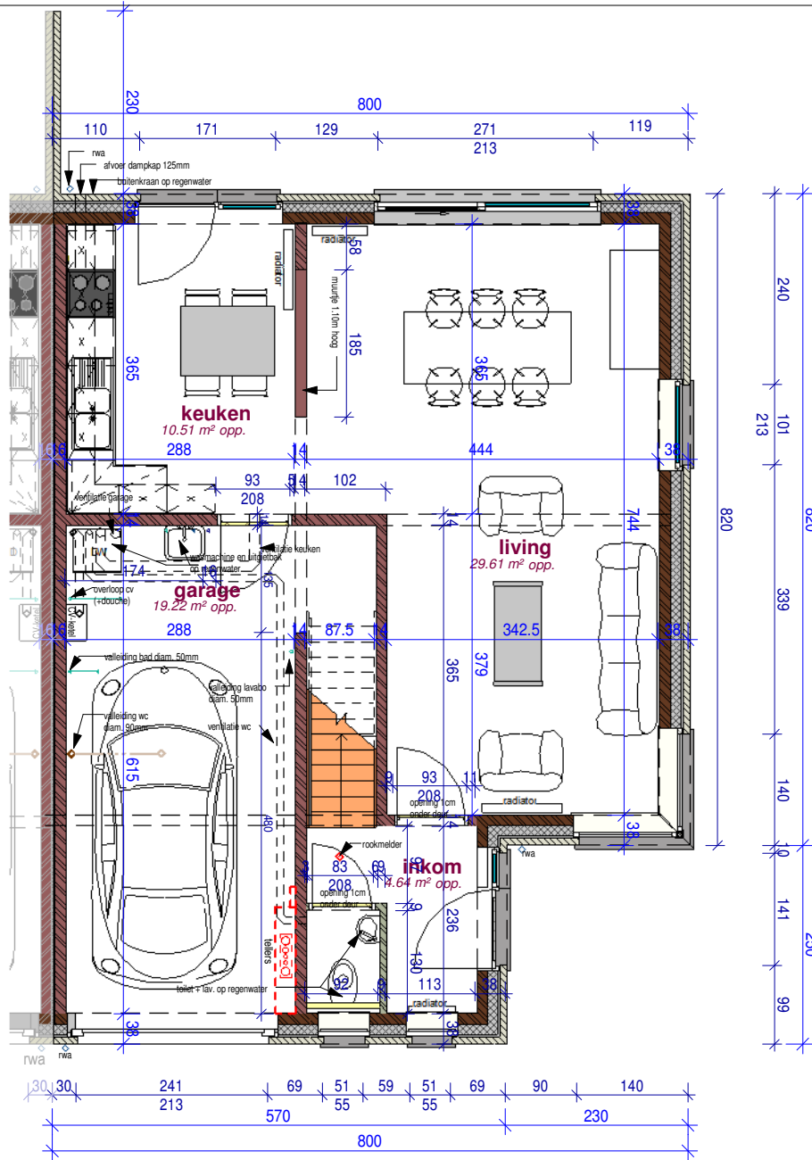
gelijkvloers
