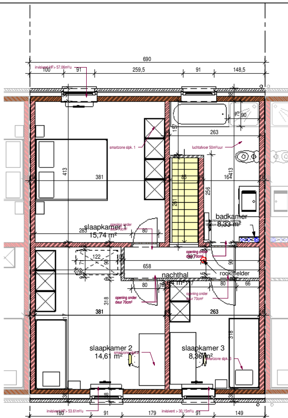
1ste verdieping
