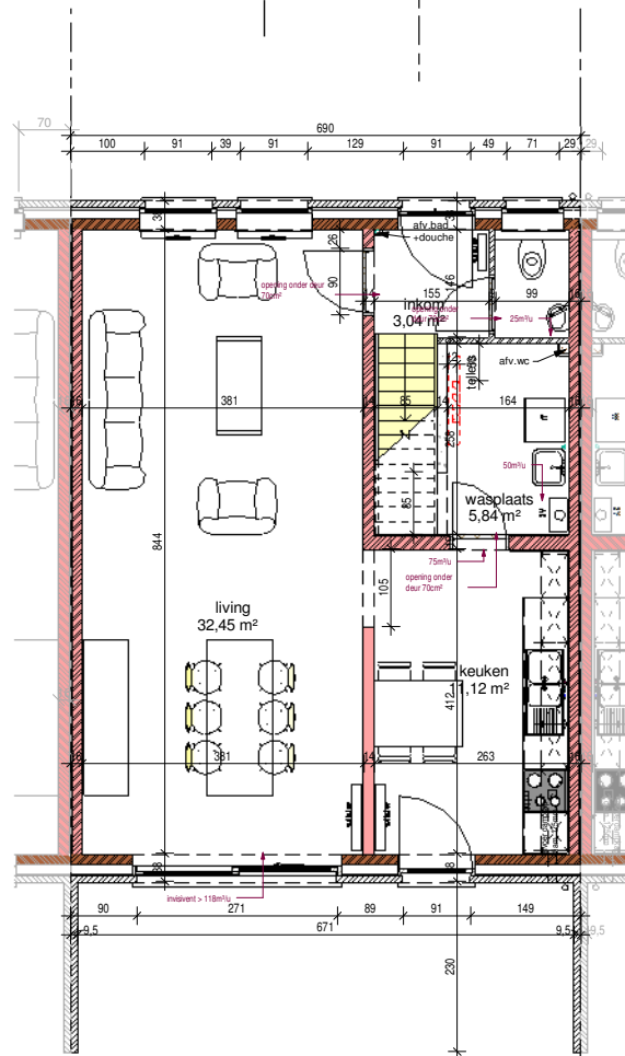
gelijkvloers
