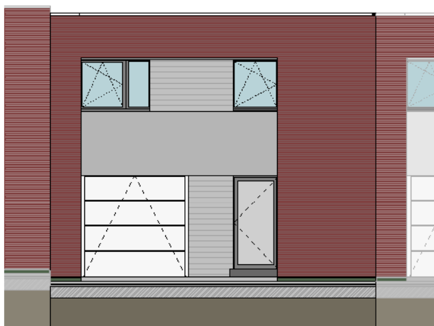
① VOORGEVEL 1 : 50
