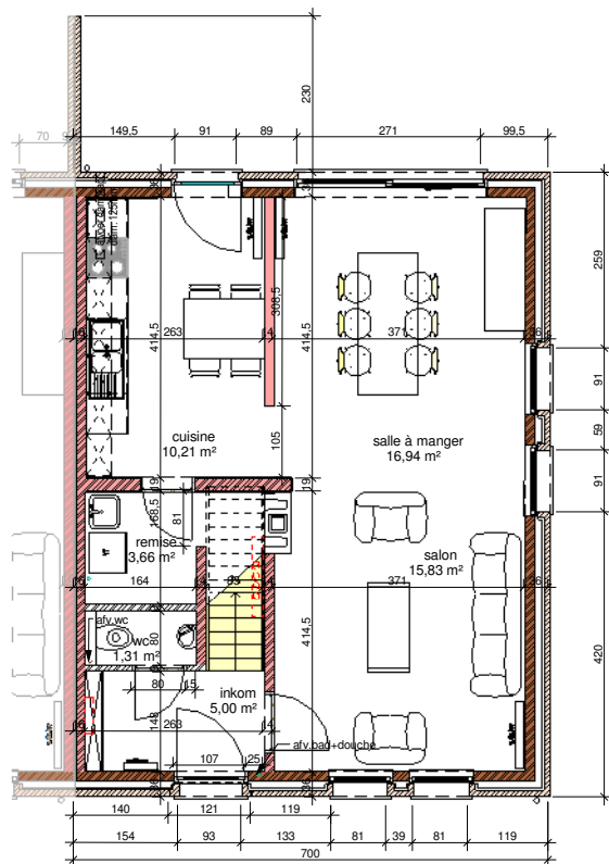
1 rez-de-chaussee 1 : 50
