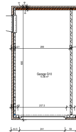
3 rez-de-chaussee, garage G10 1 : 50
