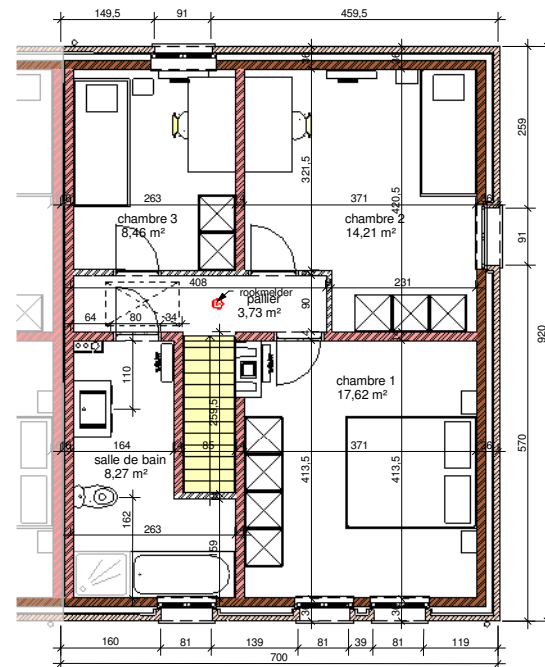
2 1° etage 1 : 50
